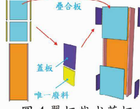
圖 4 翼板裁成蓋板 剩的腹板成疊合板
