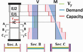
圖 2 CSPD容量設計示意圖
