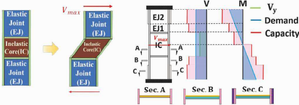
圖 1 SPD組成示意圖
