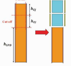
圖 3 裁切熱軋型鋼
